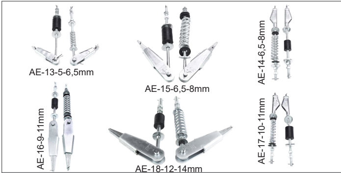
Oynar Başlıklı ve Sabit Halat Şişeleri Swinging-Fixed Rope Attachment
