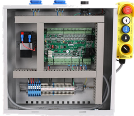
Dışısız Pano Gearless Control Panel
