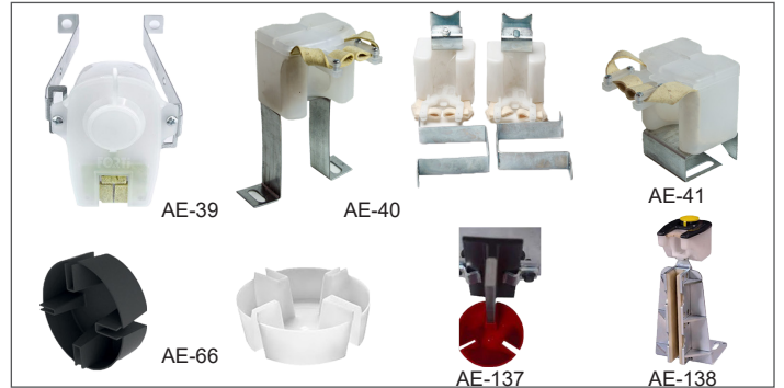
Yağdanlık Yağ Yoplama Kabı Lubricator Oil Collection Cup
