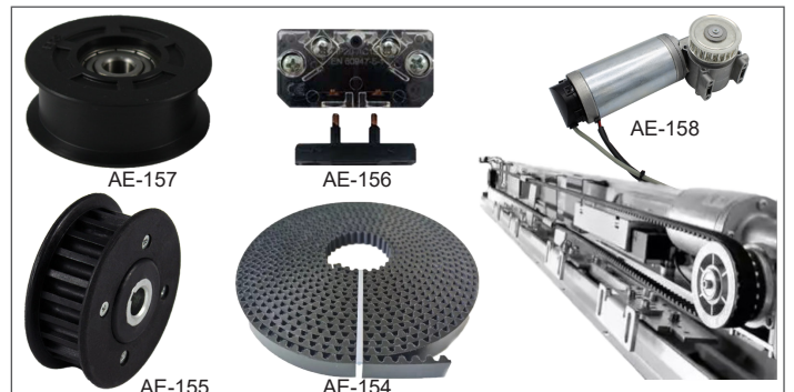
Gerdirme Kasnağı Fiş Kontakt Motor ve Dişlisi Kayış Pulley Door Contactor Motor and Engine Gear Strap
